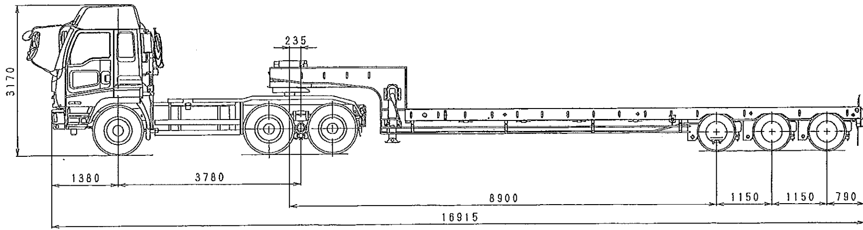
いすゞ QDG-EXZ52AJ型トラクタ 東邦 TL41KOP3S型セミトレーラ 連結状態図
